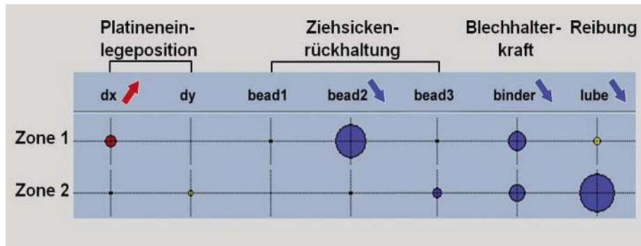
Einfluss der Korrekturmaßnahmen auf die Ausdünnung.
