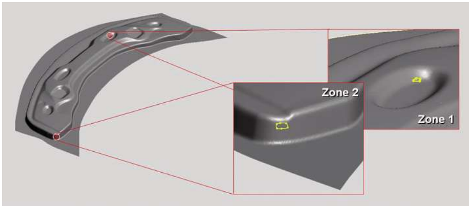
Fehler am Ziehteil während des Werkzeugtryouts. Zone 1: Riss in Verprägung, Zone 2: zu hohe Ausdünnung.
